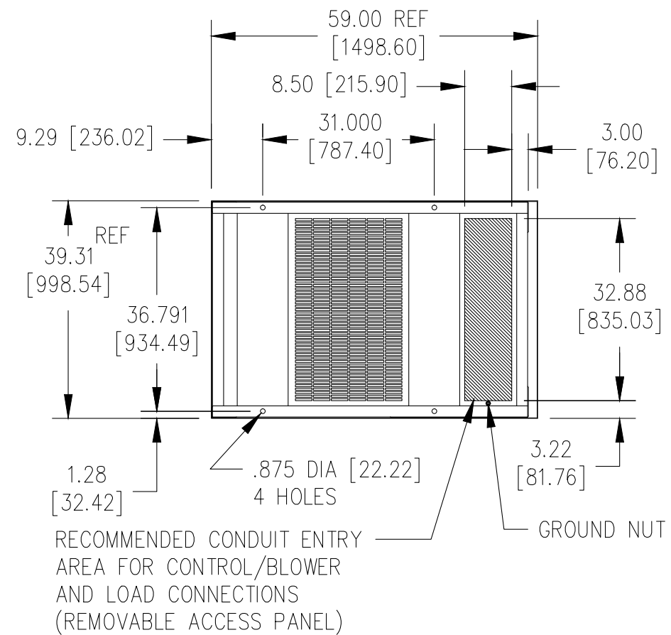
VIEW A-A
